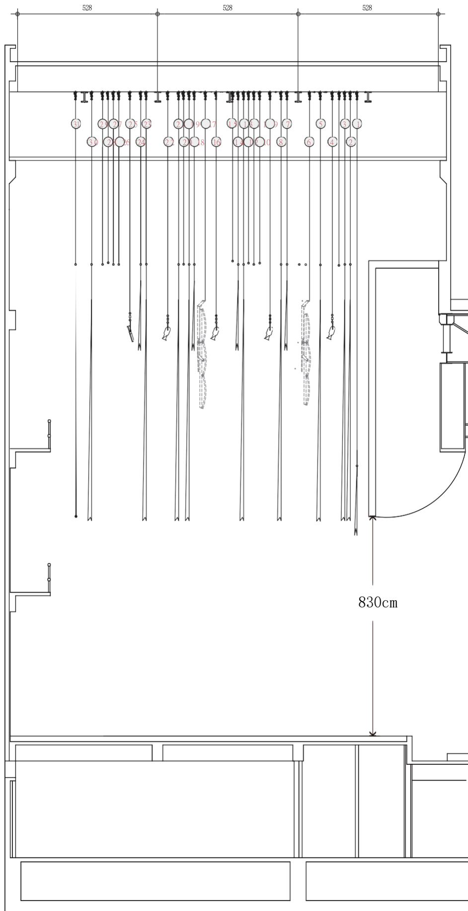
新北市藝文中心演藝廳吊具配置圖
